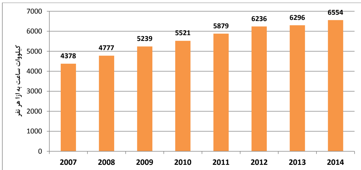
نمودار شماره ۱۹- مصرف برق در عمان طی سال های ۲۰۰۷ تا ۲۰۱۴
